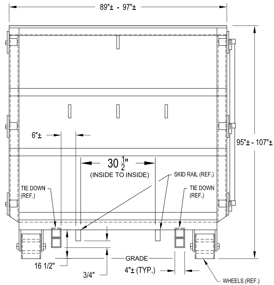
REAR VIEW SCALE: 1" = 1' (22x34) SCALE: 1" = 2' (11x17)
